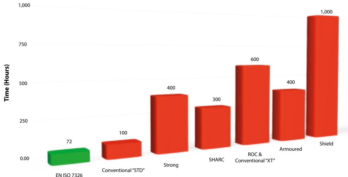
EN ISO 7326 Ozone Resistance Test
